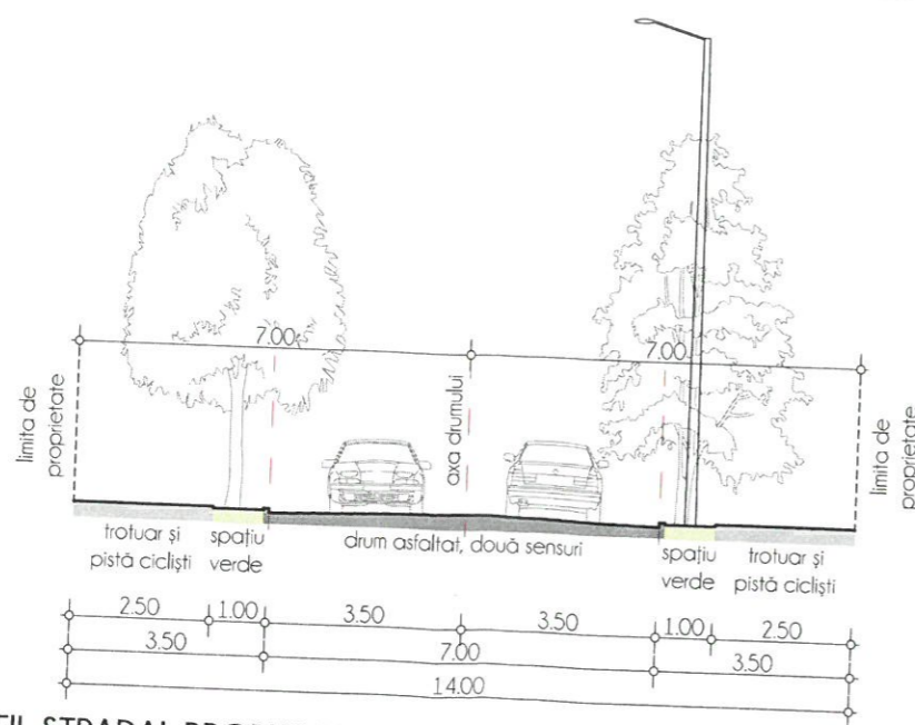
PROFIL STRADAL PROPUȘ PENTRU DRUM NR. CAD. 196036 - sc. 1:150
