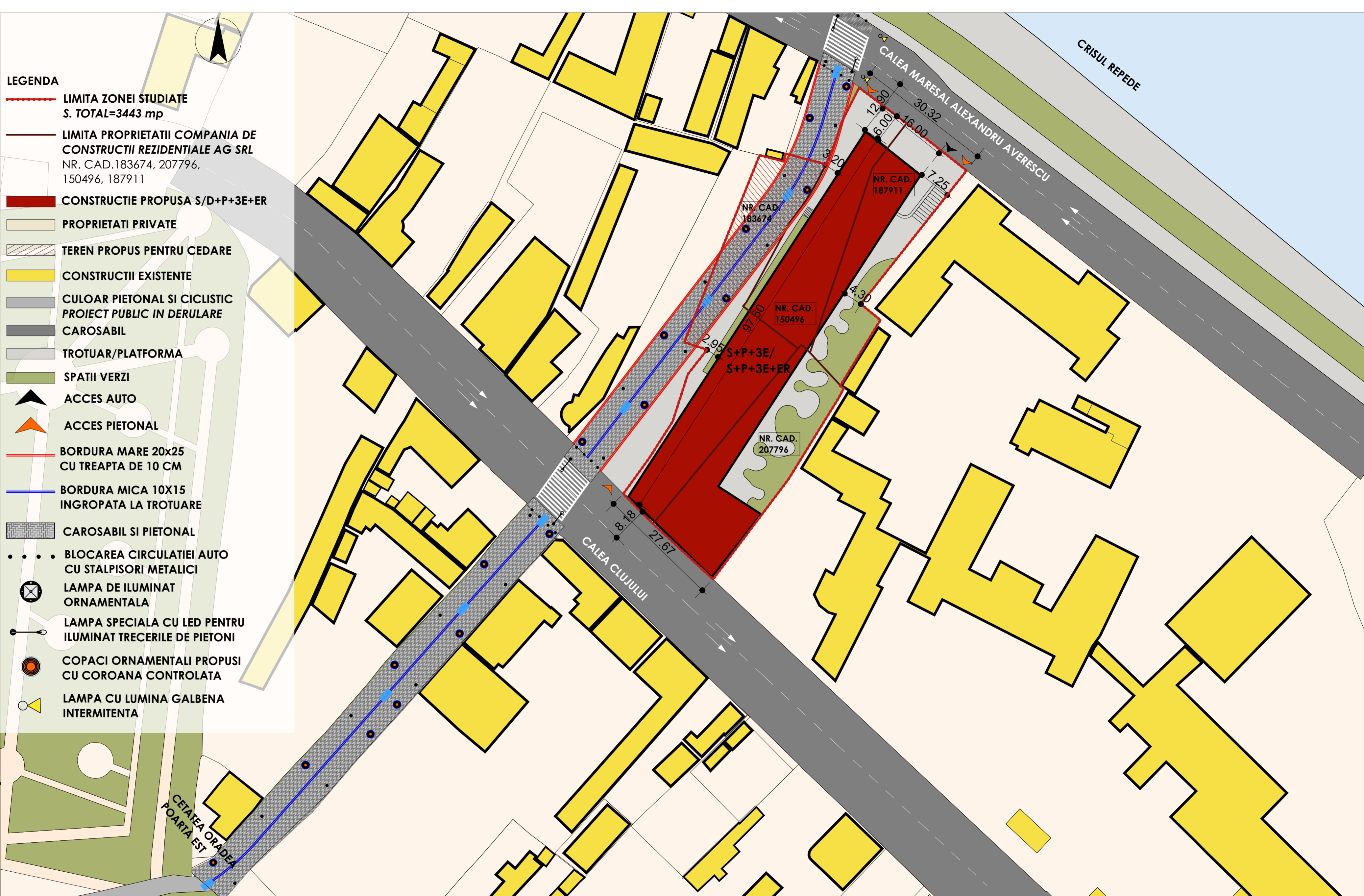
PLAN REGLEMENTARI - AMENAJARE CORIDOR PIETONAL, SC. 1:500
