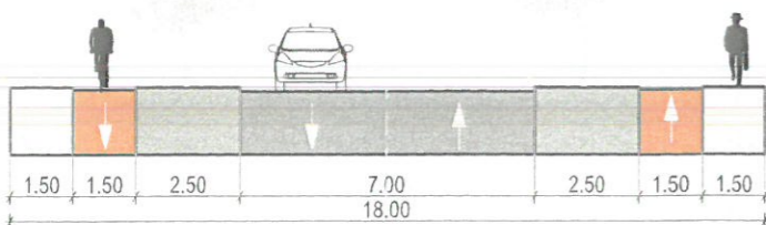
SECȚIUNE TRANSVERSALĂ DRUM CONF. P.U.G. PROFIL PROPUȘ PRIN P.U.G., SC.1:200 Str. Alexandru Macedonski
